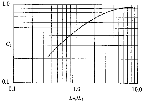
图 5.4.3 等效峰值压力系数的确定
