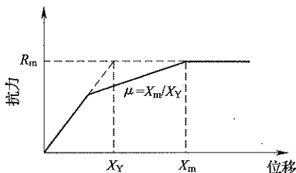
图 4 理想的位移-抗力-延性关系
