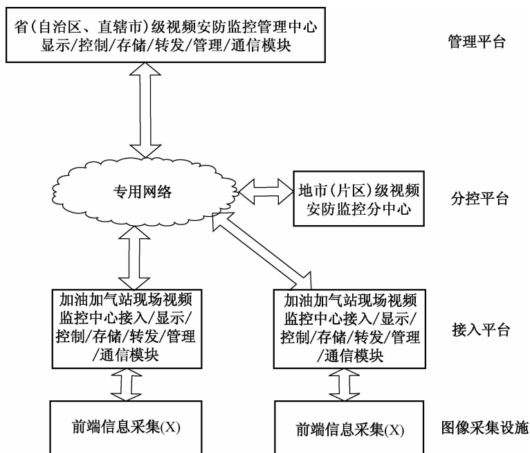
图 1 加油加气站视频安防监控系统总体架构图
