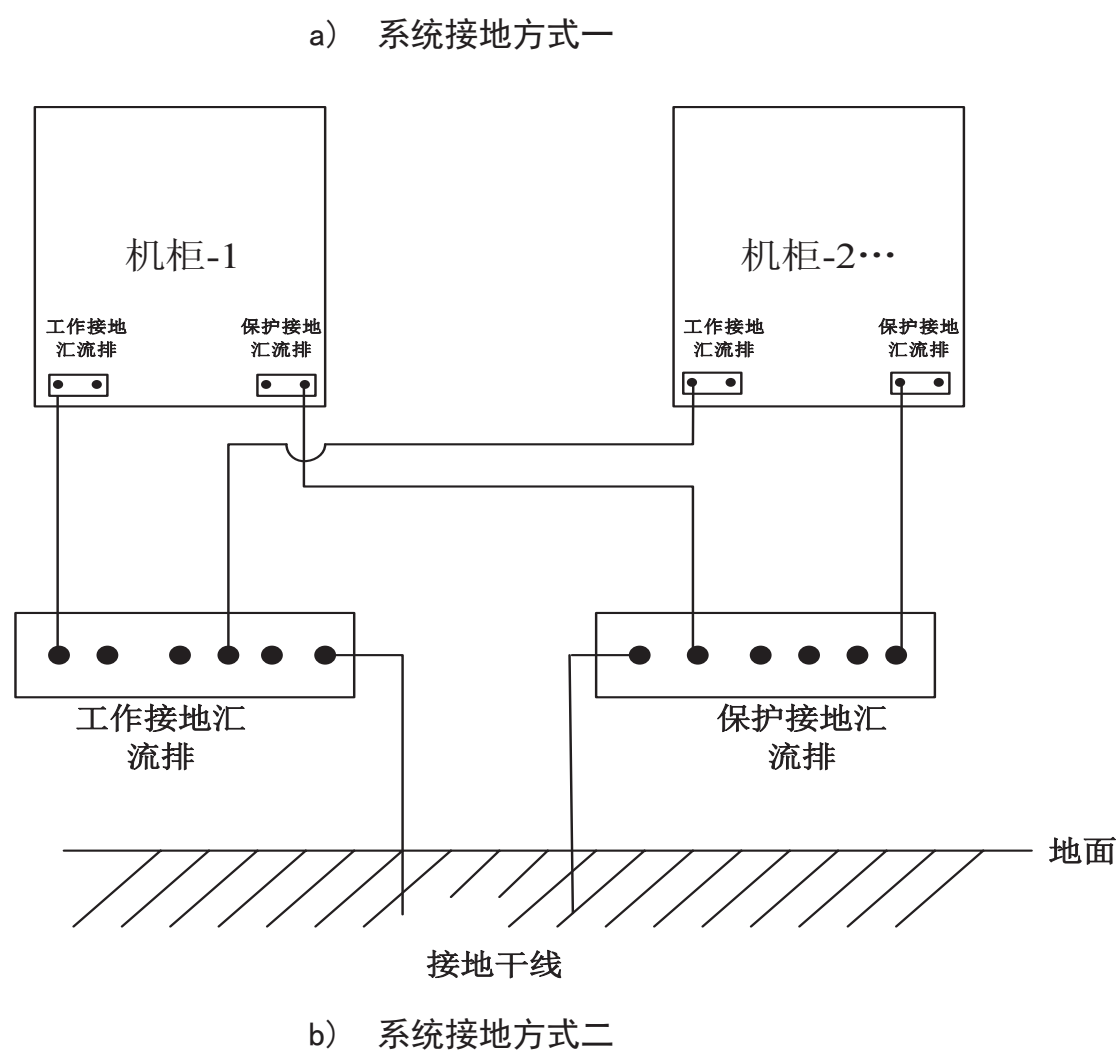
图 9.2 系统接地方式
