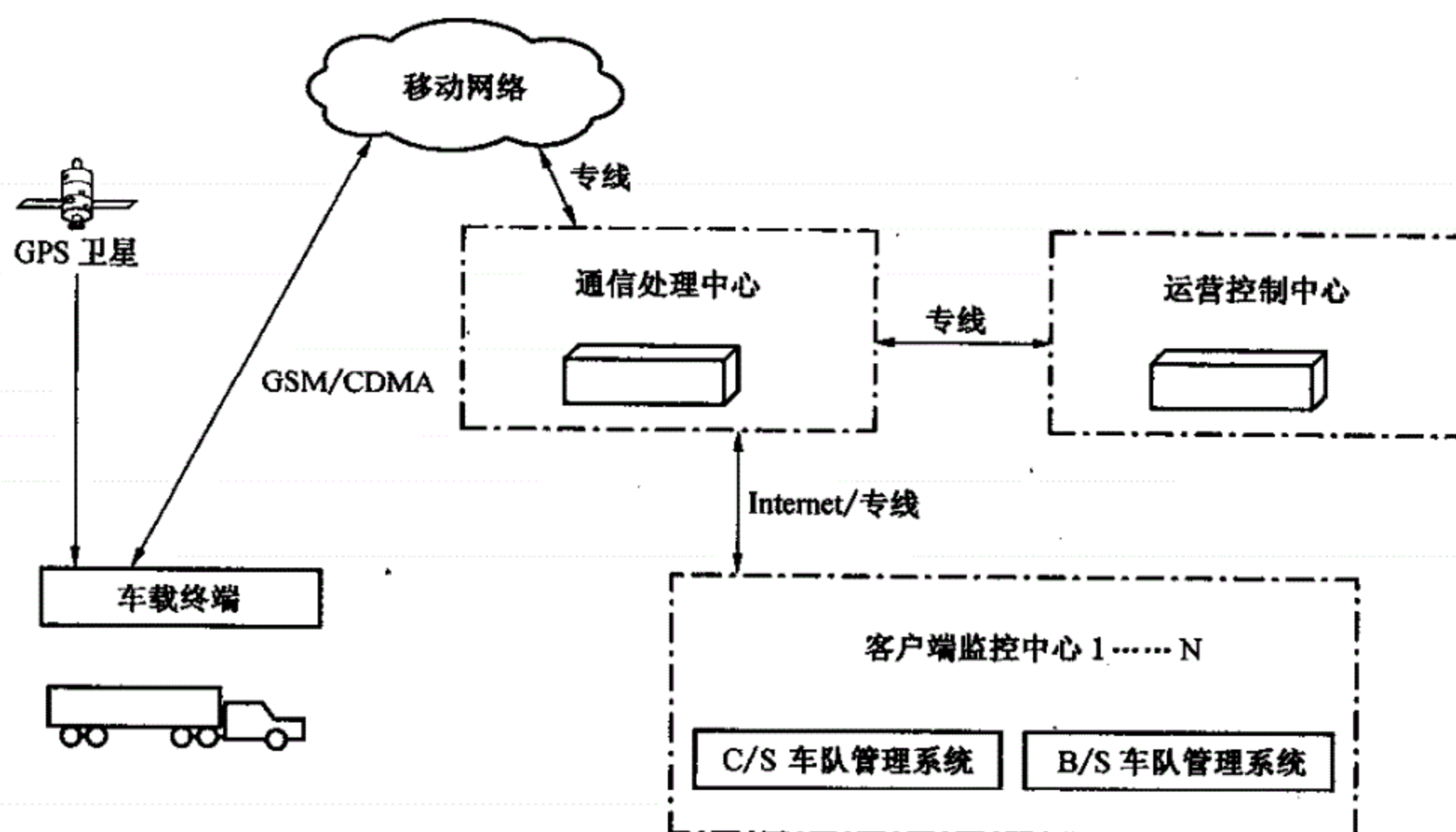
图 1 系统结构
