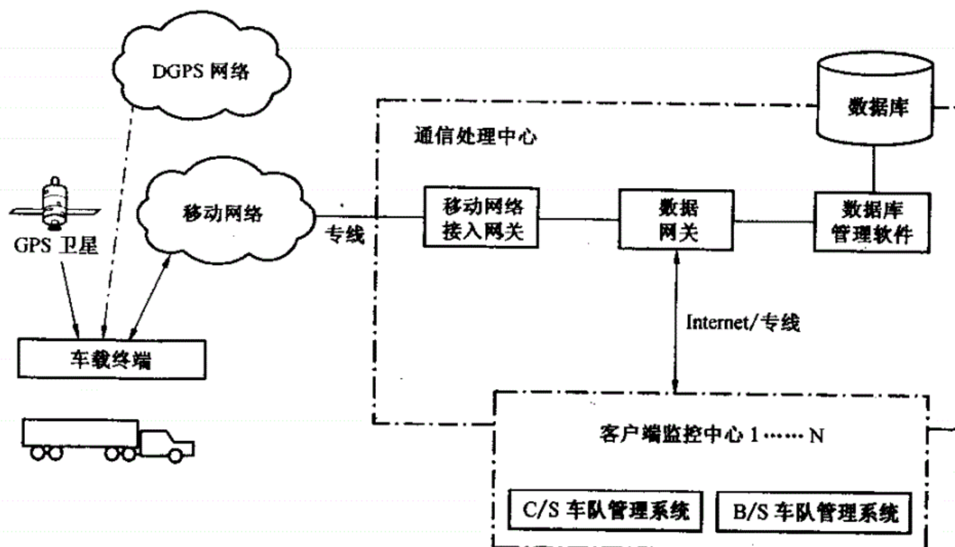
图 2 通信处理中心及接口的逻辑结构
