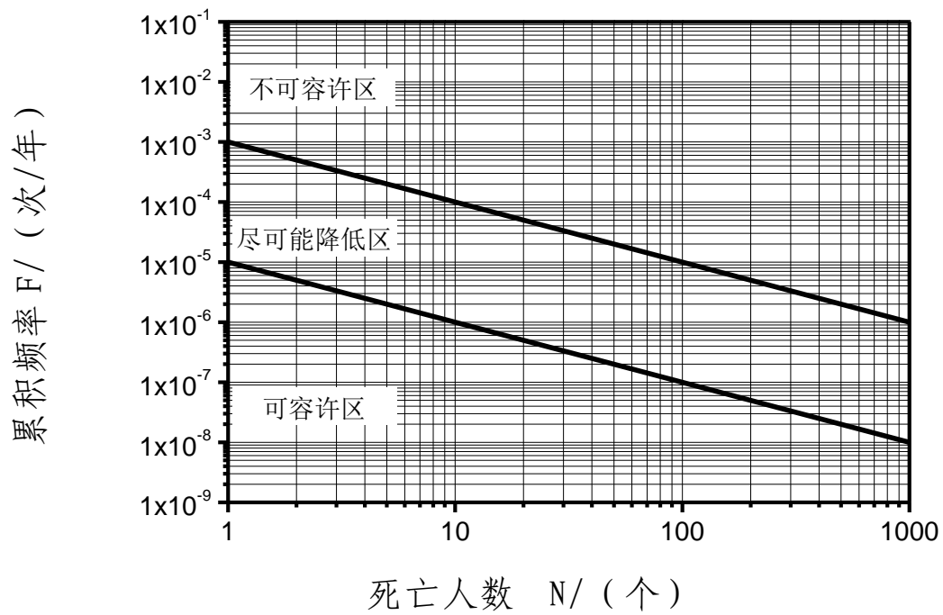
图 1 可容许社会风险标准 ( F-N ) 曲线
